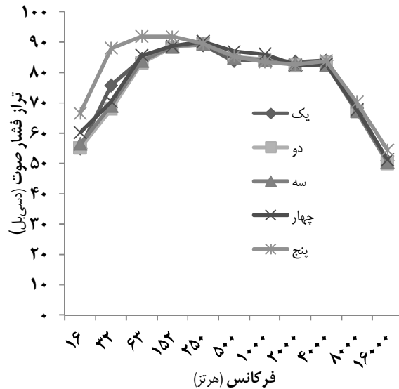
نمودار ۳) نتایج آنالیز فرکانس در موقعیت گوش راننده در دنده‌های مختلف در دور موتور ۱۷۰۰ دور بر دقیقه در تراکتور رومانی در حال حرکت
