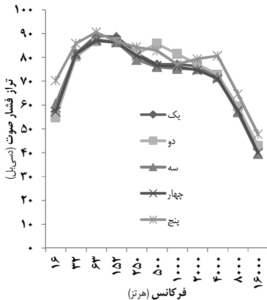
نمودار (۲) نتایج آنالیز فرکانس در موقعیت گوش راننده در دنده‌های مختلف در دور موتور ۸۵۰ در بر دقیقه در تراکتور رومانی در حال حرکت
