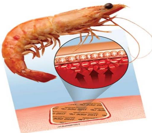
شکل-۲. Chitin polymer
